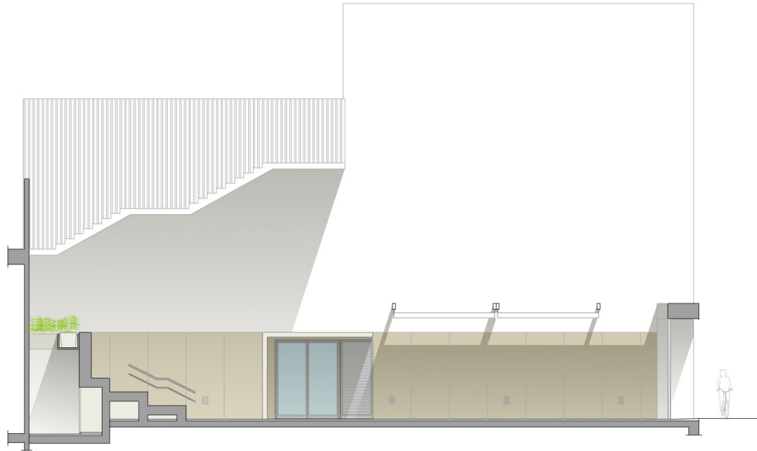
SECCIÓ LONGITUDINAL DEL NOU PATI
